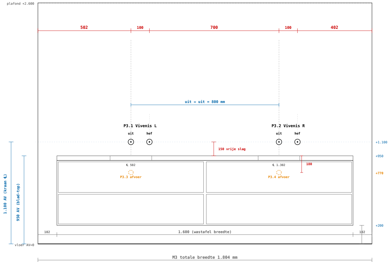
M3 – WASTAFELWAND · 2× VIVENIS · MATEN IN MM · AV VANAF AFGEWERKTE VLOER · \varnothing = HARTLIJN
